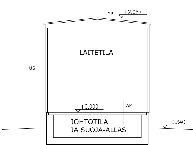
Yleisleikkaus A-A
