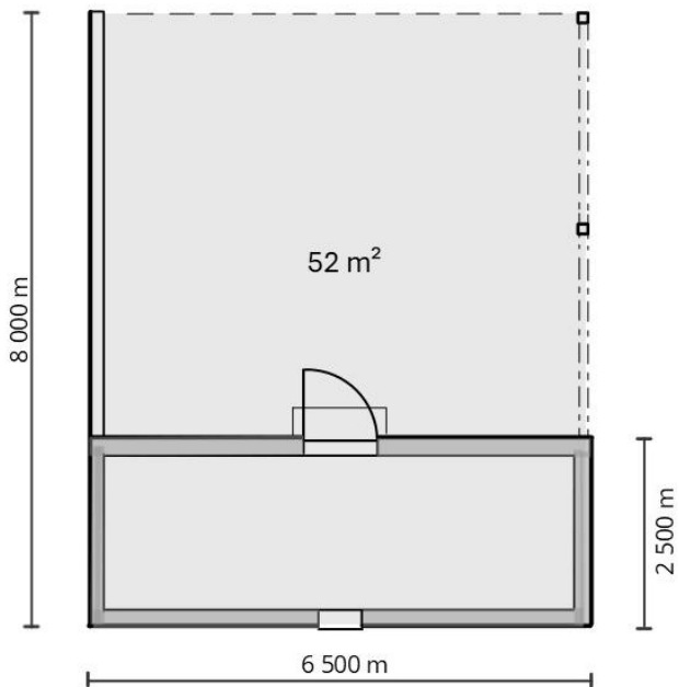
Bild 3. Exempel på beräkning av total yta
