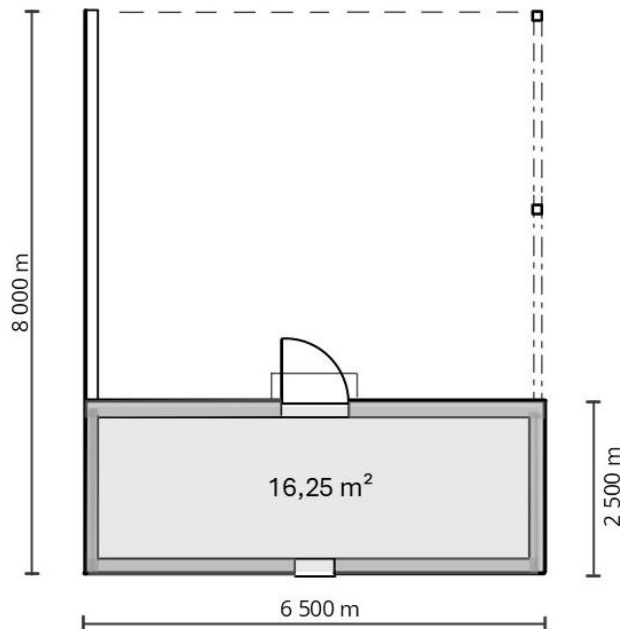
Bild 2. Exempel på beräkning av våningsyta
