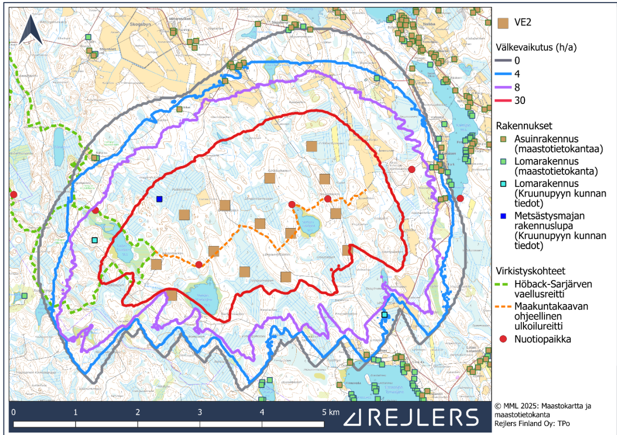
Kuva 78. Välkemallinnus hankevaihtoehdolle VE2 (Rejlers Finland Oy).
