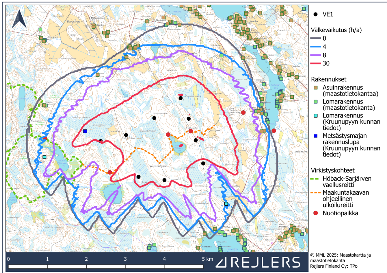
Kuva 76. Väkemallinnus hankevaihtoehdolle VE1 (Rejlers Finland Oy).
