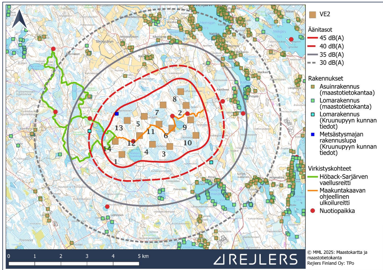
Kuva 75. Melumallinnus hankevaihtoehdolle VE2 (Rejlers Finland Oy).
