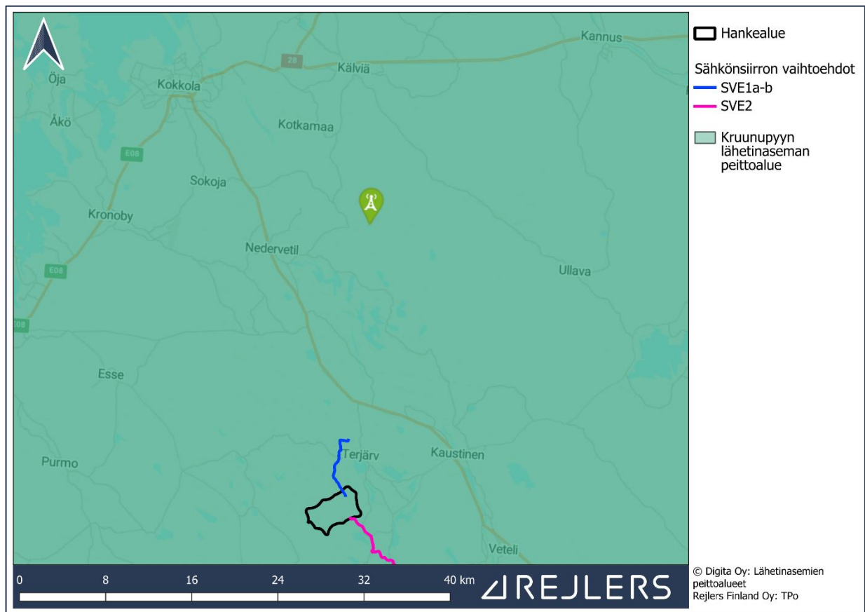
Kuva 87. Digitan Kruunupyyn lähetaseman näkyvyyskartta. Kruunupyyn lähetaseman sijainti on esitetty kartalla vihreällä pisaralla.
