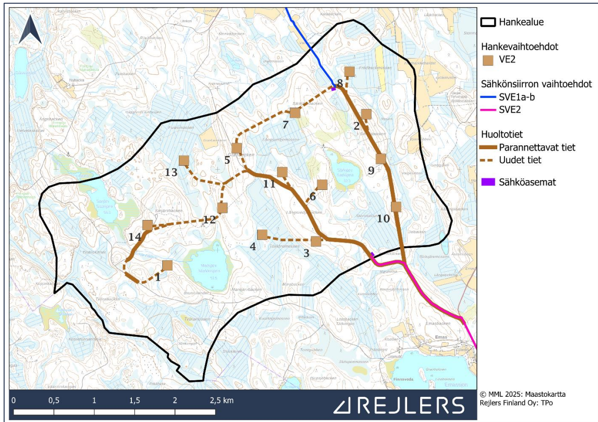
Kuva 4. Voimalasijoittelu hankevaihtoehdossa VE2.
