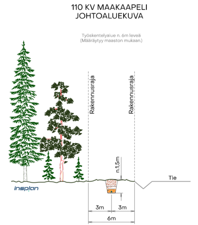
Kuva 8. Reittivaihtoehdoissa SVE1a ja SVE2 käytettävän 110 kV:n maakaapelin johtoaukean poikkileikkaus (Insplan Oy).
