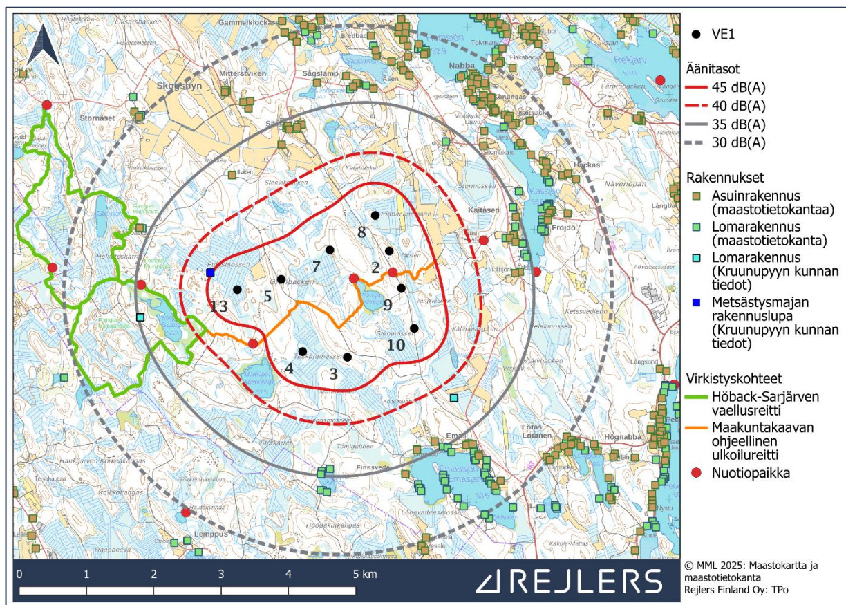
Kuva 73. Melumallinnus hankevaihtoehdolle VE1 (Rejlers Finland Oy).
