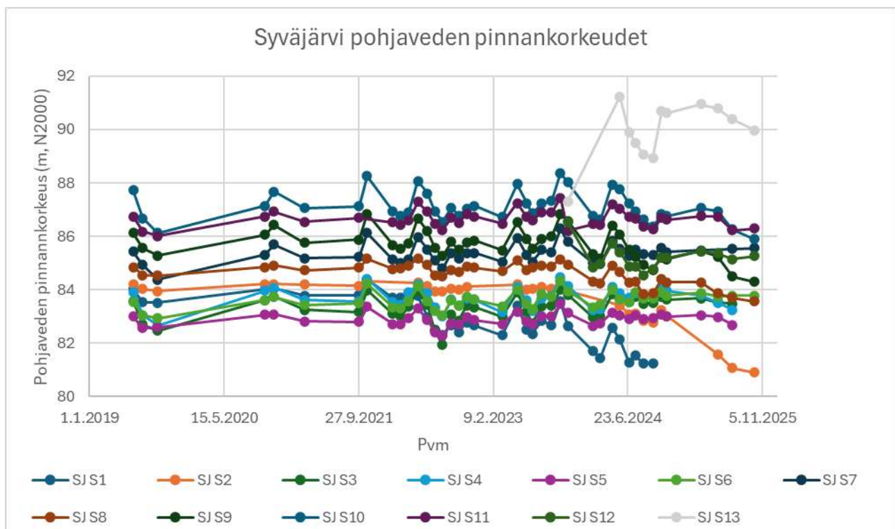
Kuva 3-2. Syväjärven pohjavesiputkien tarkkailutulokset vuosina 2019–2025.
